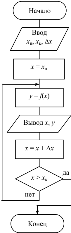
Рис. 6. Блок-схема алгоритма табулирования функции (циклический алгоритм)
