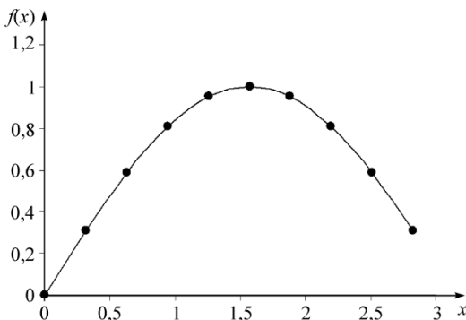
Рис. 26. Построение интерполирующей функции по дискретному набору исходных табличных данных: ● – исходные табличные данные; — интерполирующая функция f(x)
